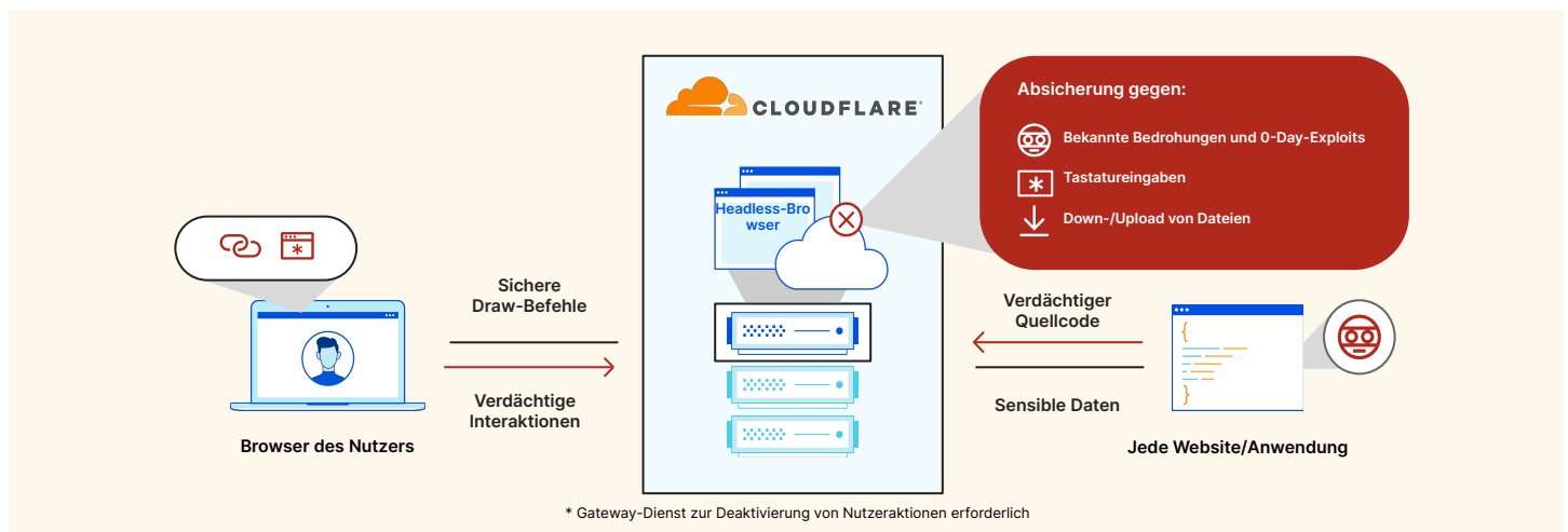
Abbildung 2: Isolierte Sitzung
