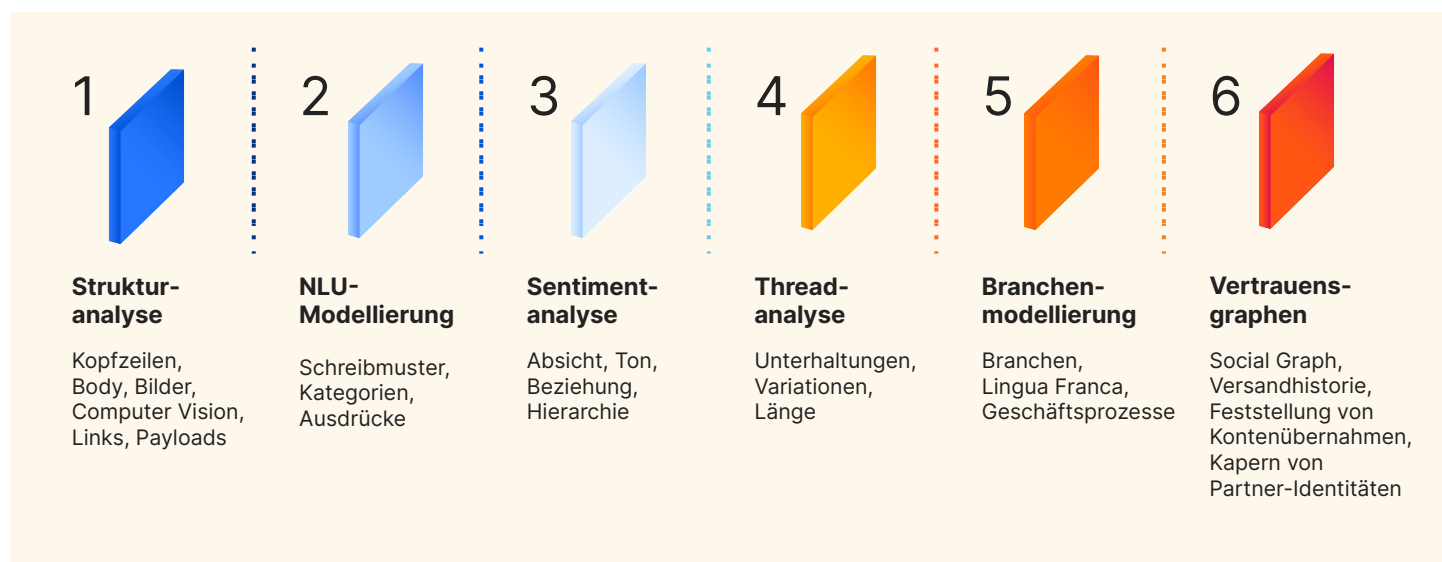
Abbildung 1: Nachrichtenanalyse
